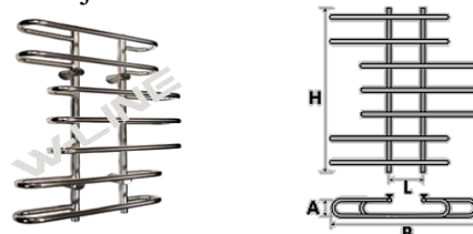
Dvieļu žāvētājs "SAIL"
